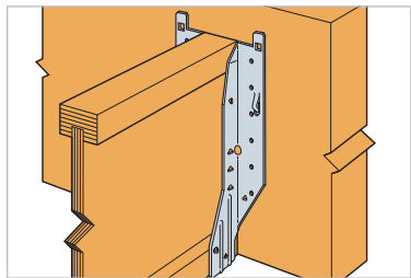
Типичная установка IUSE.
