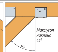
LBV возможная дополнительная установка
