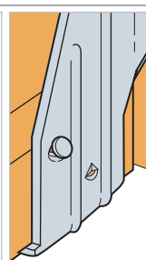
Типичное выполнение узла с применением опоры ITSE: соединитель крепится к несущей стальной двутавровой балке с помощью деревянной планки.
