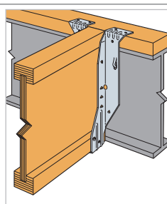
Типичное выполнение узла с применением опоры ITSE: соединитель крепится к несущей стальной двутавровой балке с помощью деревянной планки.
