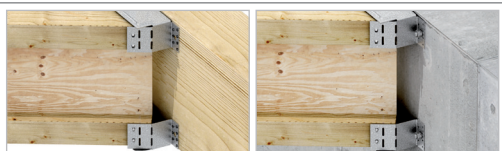
Вид соединения дерево/дерево
