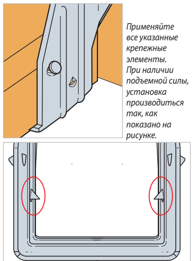
Типичная установка IUSE.
