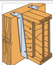
LBV Типичная установка
